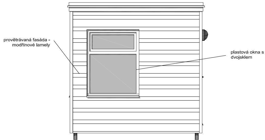
POHLED ZÁPAD
