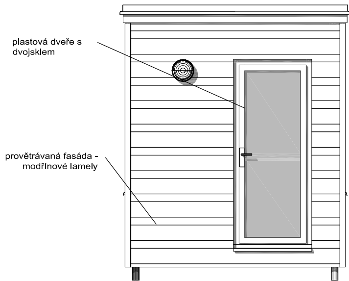
POHLED SEVER
