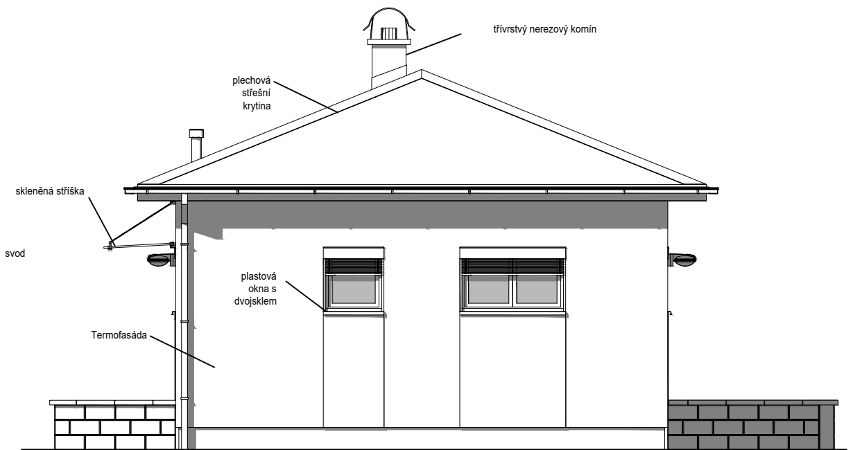
POHLED ZÁPAD
