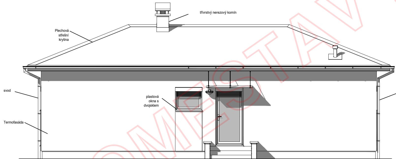
POHLED SEVER
