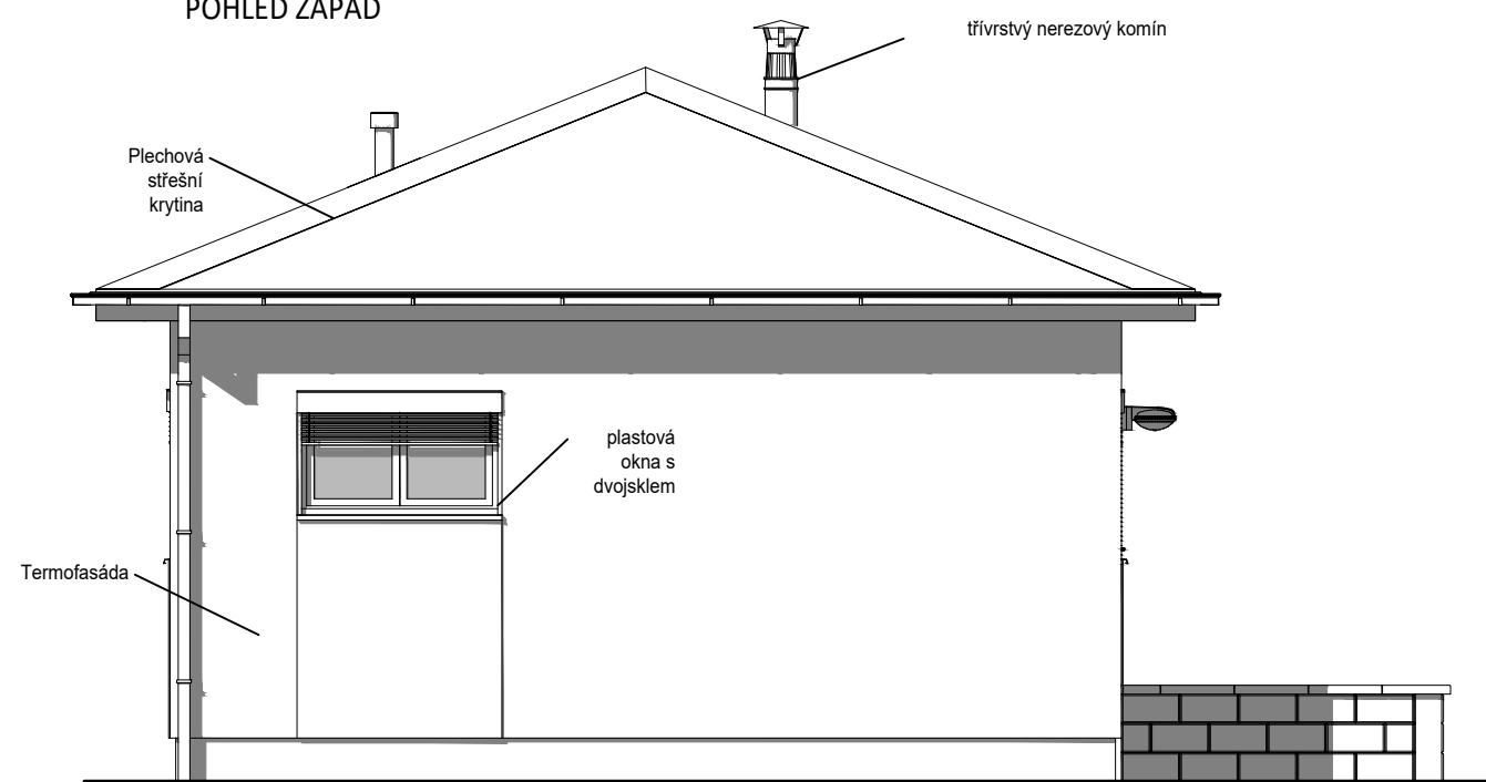
POHLED ZÁPAD
